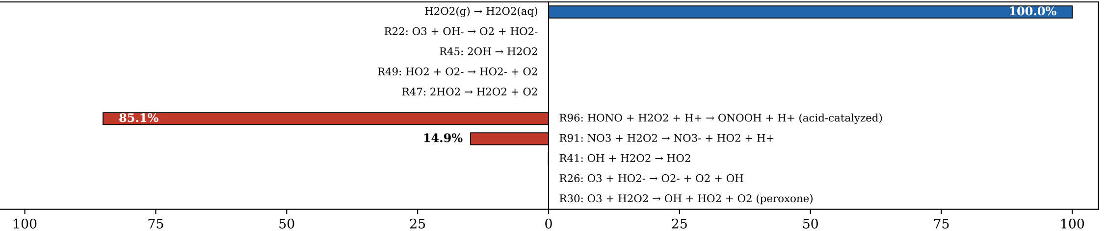
(d) H 2 O 2 (Σsrc = 1.06e-08 M/s)
